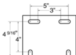
Mounting Plate (GBA-642, GBA-542)
